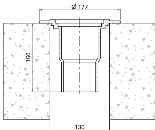
Balkoninė, Tipas A 50/70 vertikali
