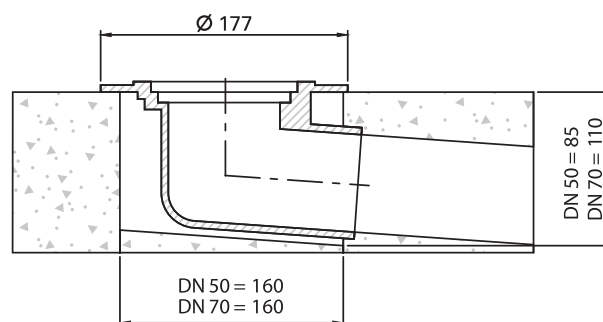
Balkoninė, Tipas A, horizontali
