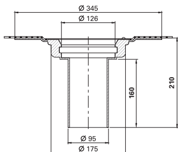
Kingspan ESSMANN DN 95 renovacinė įlaja, su užv. žiedu
