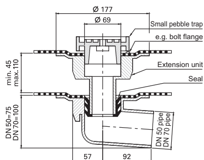
Kingspan ESSMANN balkoninė įlaja DN 50 ir DN 70 horizontali
