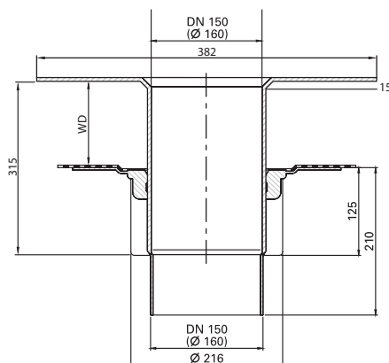
DN 150 Vertikali užveržiamo žiedo
