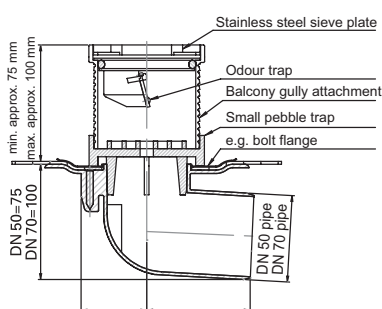
Kingspan ESSMANN balkoninė įlaja su apsauga nuo kvapų
