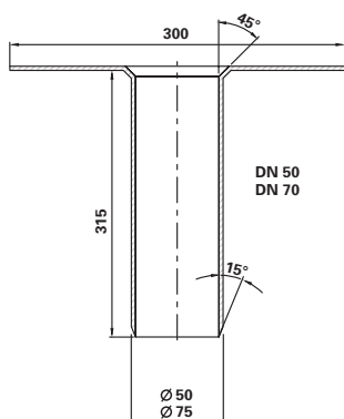
Kingspan ESSMANN DN 50/70 Classic renovacinė įlaja 2
