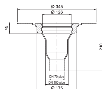
Kingspan ESSMANN kintamo ilgio įlaja, su užv. žiedu
