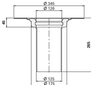
Kingspan ESSMANN DN 125 renovacinė įlaja, su užv. žiedu
