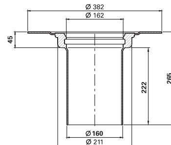
Kingspan ESSMANN DN 165 renovacinė įlaja, su užv. žiedu
